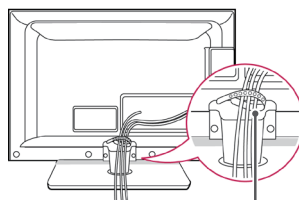
Držák kabelů
